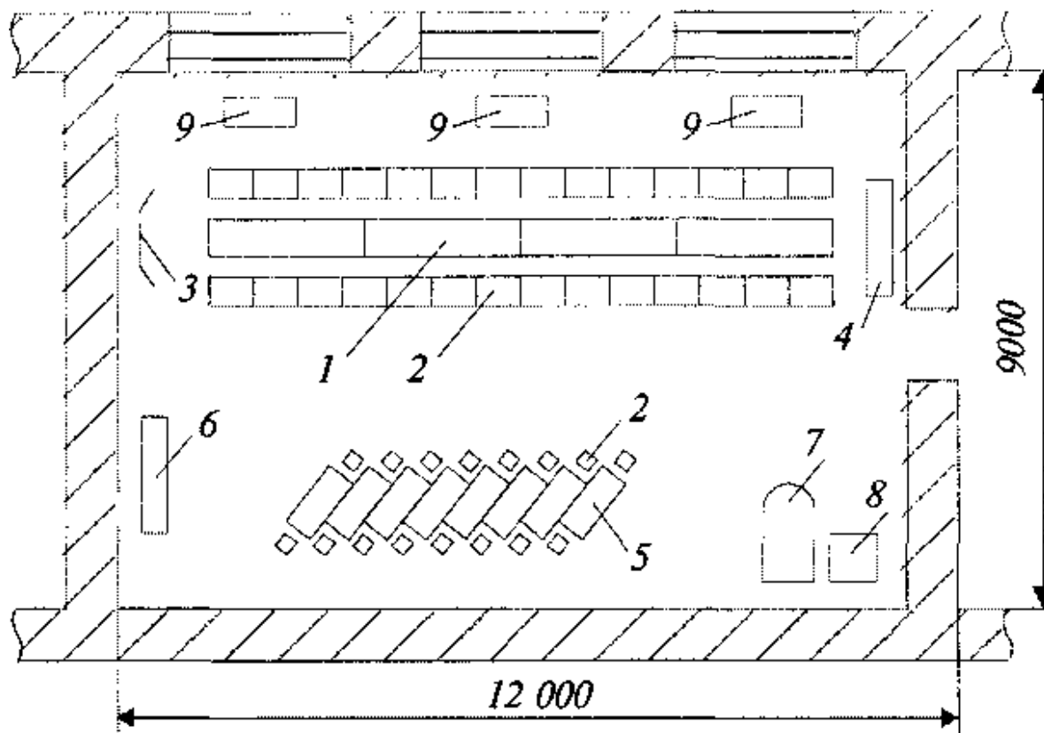
Рис. 11.2. Типовая планировка комнаты совещаний и деловых встреч: 1 — стол для совещаний; 2 — стулья; 3 — экран; 4 — шкаф для проекционной аппаратуры; 5 — столы для совещаний; 6 — шкаф для макетов; 7 — стол журнальный; 8 — кресло для отдыха; 9 — цветочница
