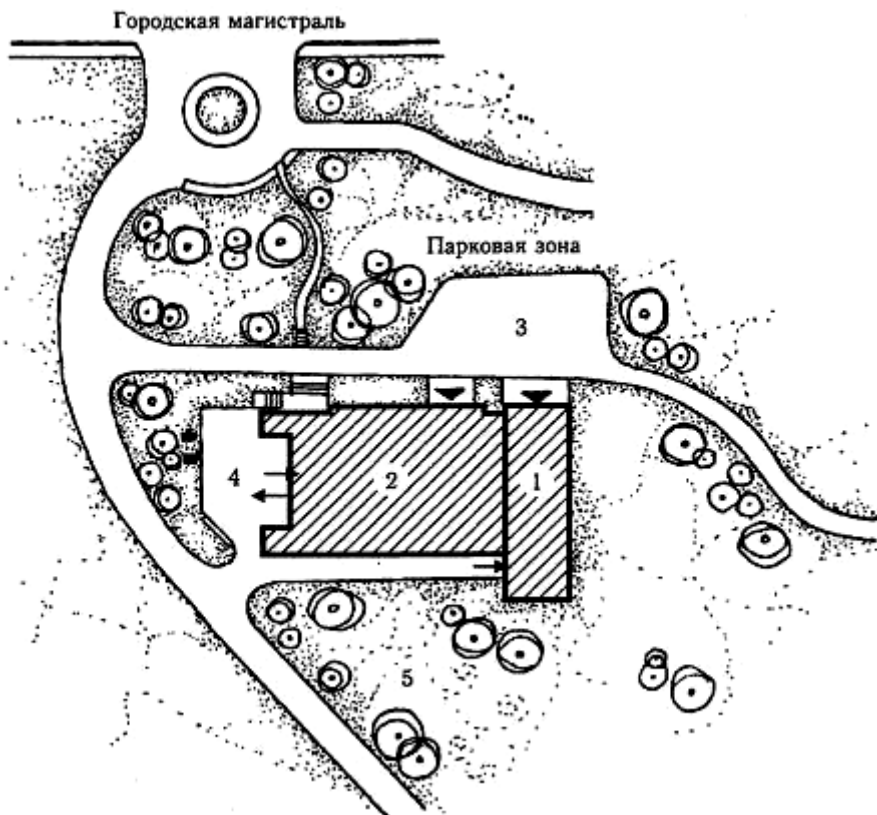
Рис. 3.17. Планировочная организация территории городской гостиницы: 1 — жилой корпус; 2 — то же, общественно-административный; 3 — автостоянка; 4 — хозяйственный двор; 5 — зеленая зона
