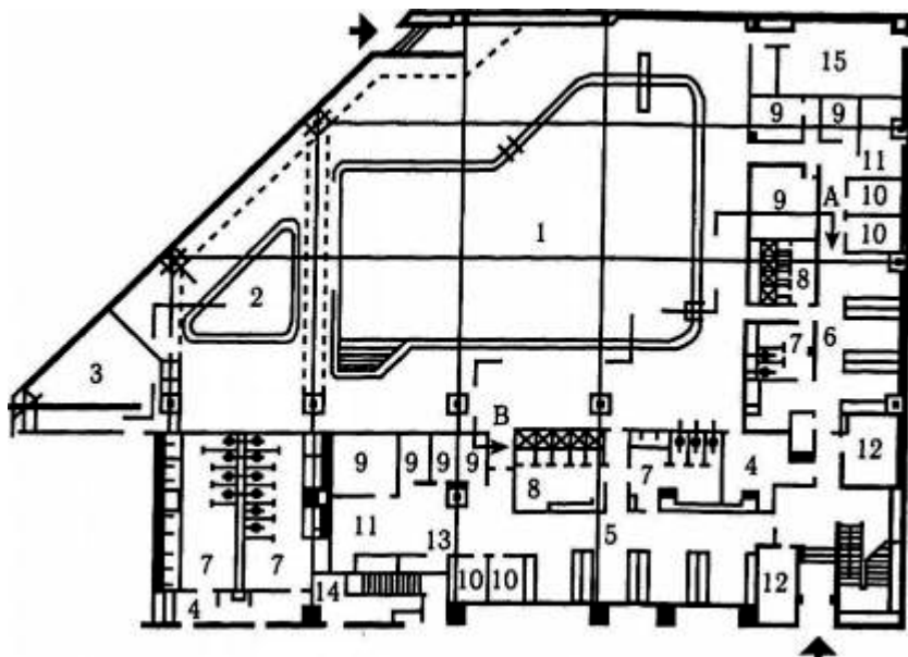
Рис. 4.24. Планировочная организация спортивно-оздоровительных учреждений: 1 — плавательный бассейн; 2 - то же, плескательный; 3 - закусочная; 4 — медпункт; 5 — мужская раздевальня; 6 — то же, женская; 7 — туалет; 8 — душевая; 9 - сауна; 10 — массажная; 11 — комната отдыха; 12 — комната выдачи полотенец; 13 — кладовая; 14 — тамбур; 15 - техническое помещение
