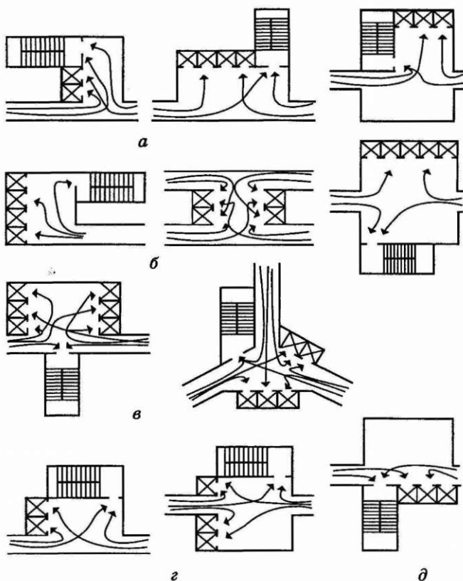
Рис. 4.13. Планировочное решение поэтажных холлов гостиницы:
