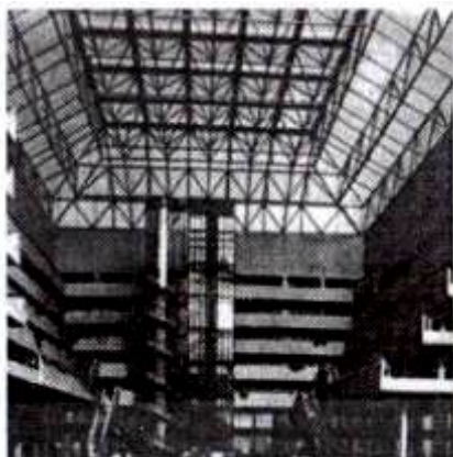
Рис. 1.48. Атриумная гостиница «Ридженс-Хайатт» (США): а — интерьер вестибюля; б — разрез; в — план
