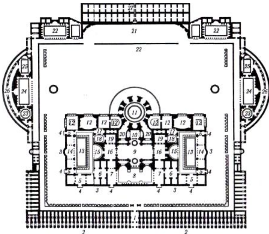
Рис. 1.6. Термы Каракаллы (Древний Рим):
