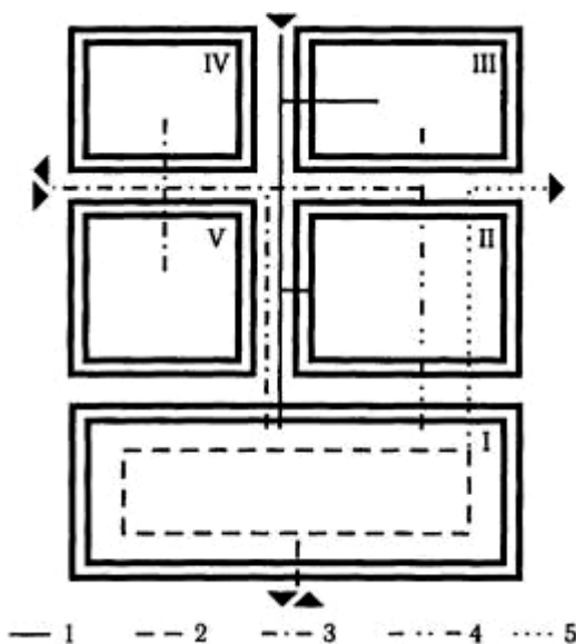
Рис. 4.18. Функциональные и технологические связи групп помещений питания:
