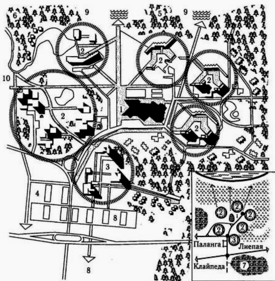
Рис. 2.24. Схема планировочной организации рекреационного поселка Ванагуге: 1 — общественный и спортивный центры; 2 — комплексы отдыха; 3 — туристские комплексы; 4 — центральная автостоянка личных и экскурсионных машин; 5 — лесопарк; 6 — парк лечебной физкультуры и климатотерапии; 7 — парк развлечений; 8 — пешеходная дорога в парк развлечений; 9 — то же, на море; 10 — то же, в Палангу
