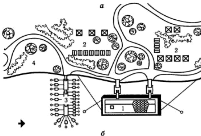
Рис. 3.28. Зонирование участка флотеля и флотокемпинга:
