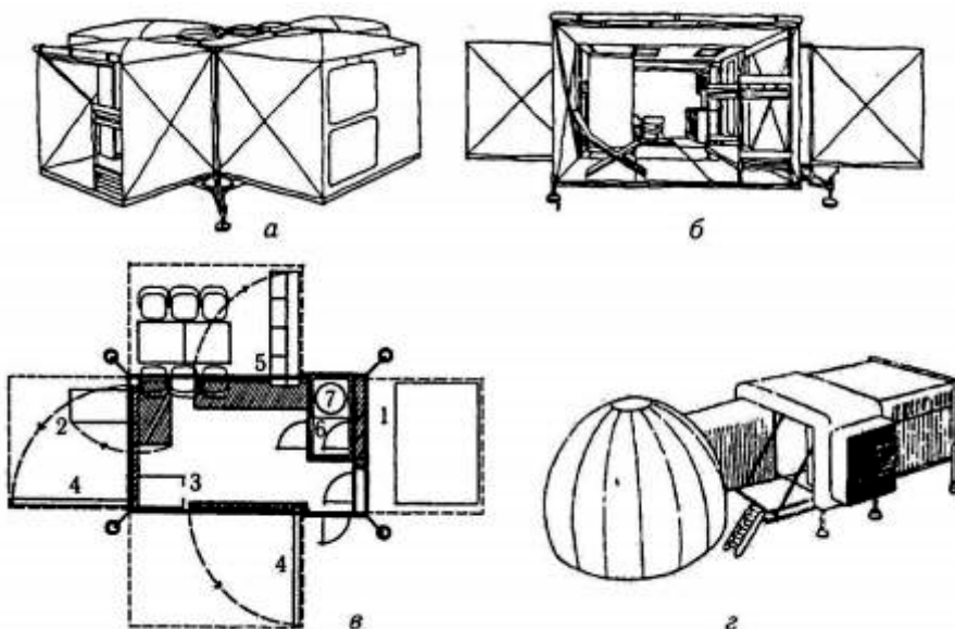
Рис. 3.36. Мобильные спальные ячейки для туристских лагерей:
