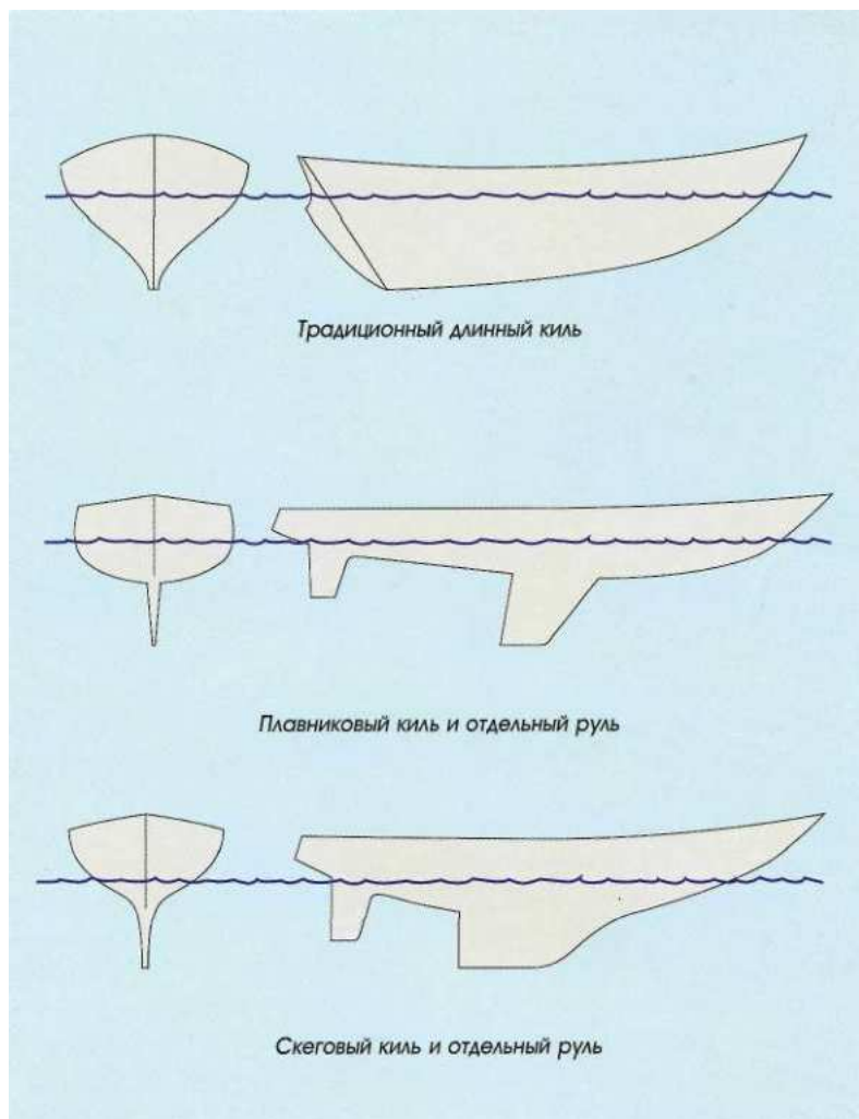
Форма киля и тип корпуса варьируются в зависимости от назначения судна. В некоторых крейсеров широкий корпус с минным глубоким килем (вверху) для надежной остойчивости, а гоночные яхты (внизу) имеют узкий корпус, позволяющий скользить по воде
