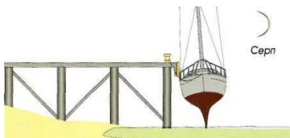
Сизигийные приливы: Солнце и Луна притягивают воду одновременно в полнолуние и при серпе; прилив в эти дни бывает самым высоким, а отлив - самым низким.
