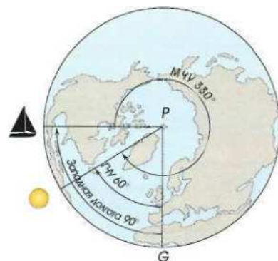
Соотношение между местным часовым углом (МЧУ), ГЧУ и долготой. МЧУ может быть восточным 30° или западным 330°
