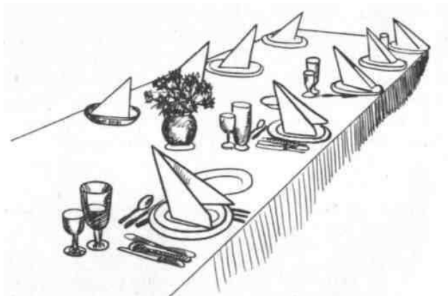
Рис. 56. Банкетний стіл
