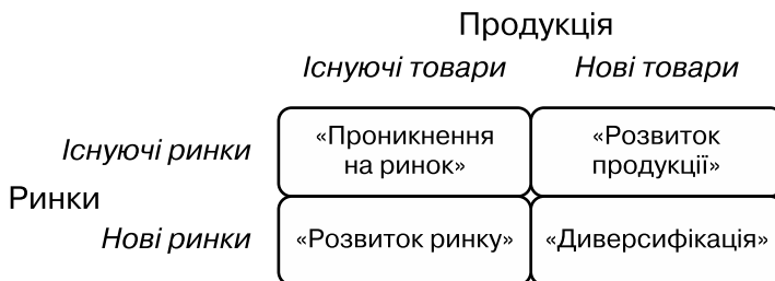
Рис. 4.12. Матриця Ансоффа
